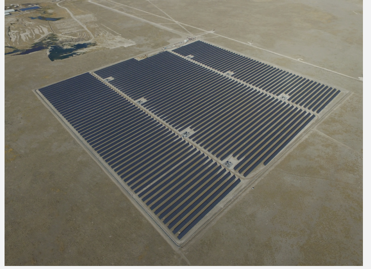
Polat Enerji Lisanslı, Cingilli GES, 36.40 MW, Niğde
